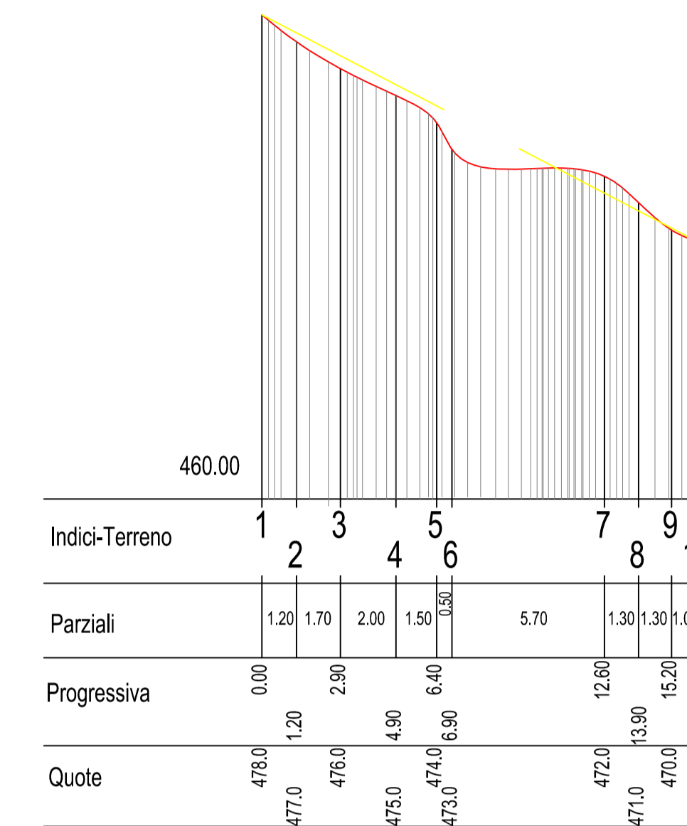
Sezione 5
