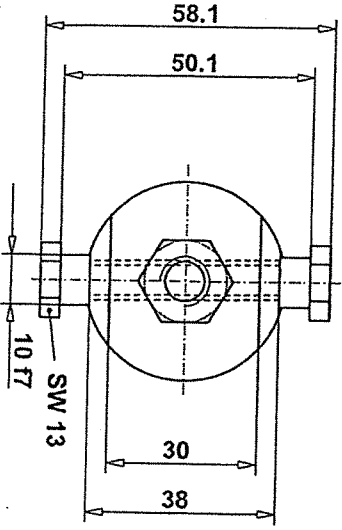
Ansicht A
