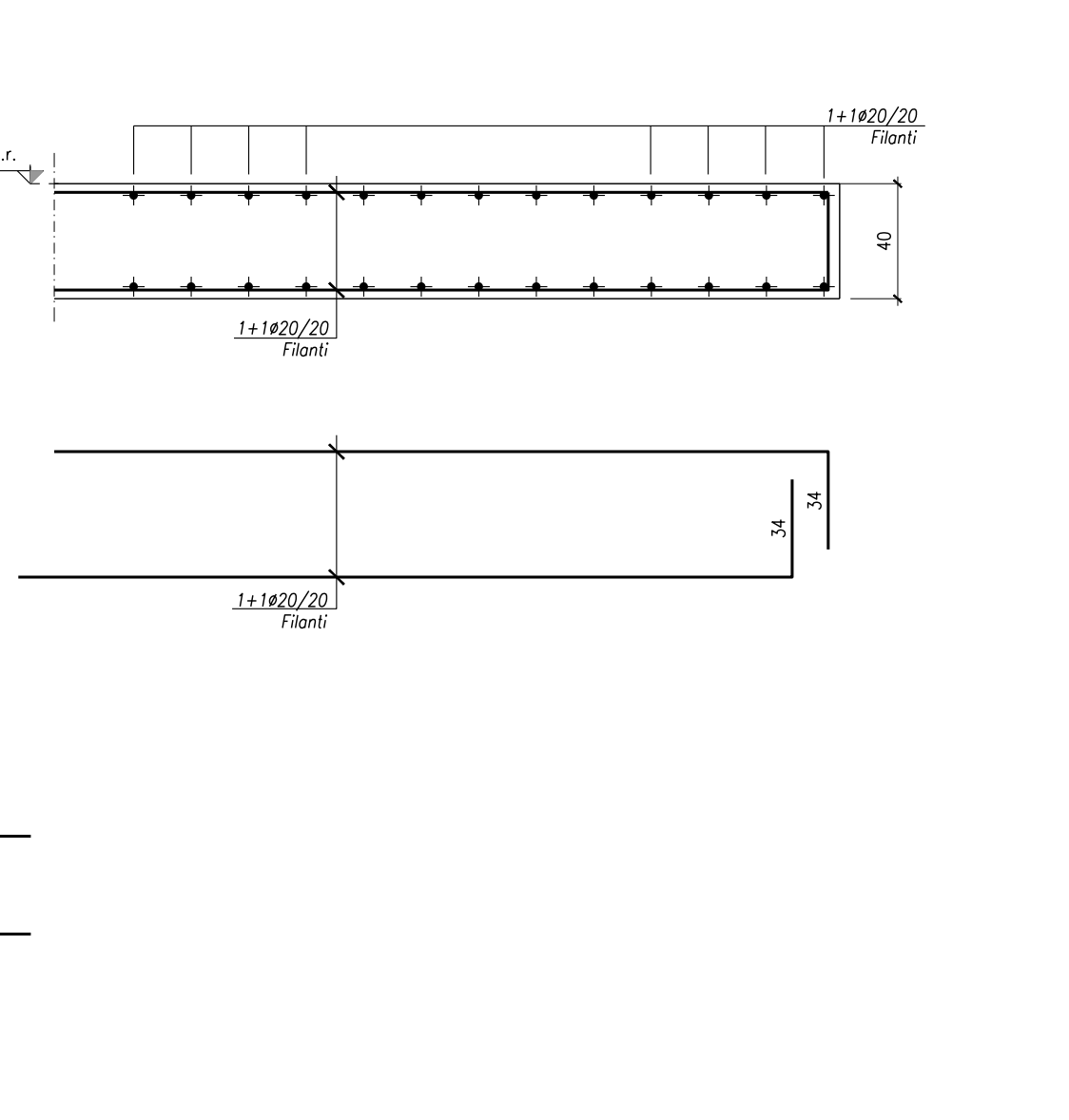
SEZIONE 4-4 SCALA 1:25
