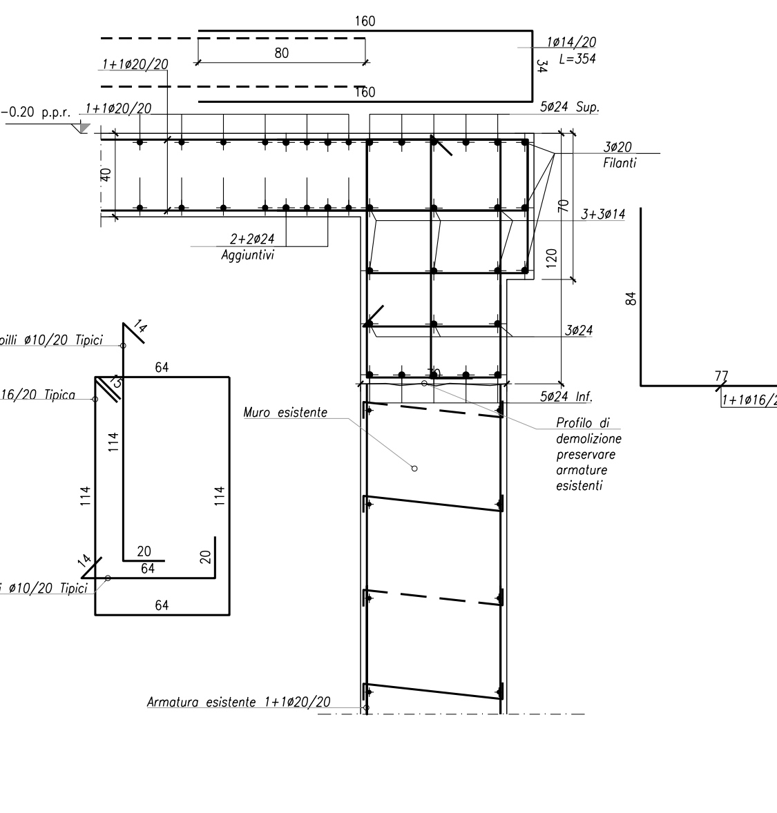
SEZIONE 2-2 SCALA 1:25
