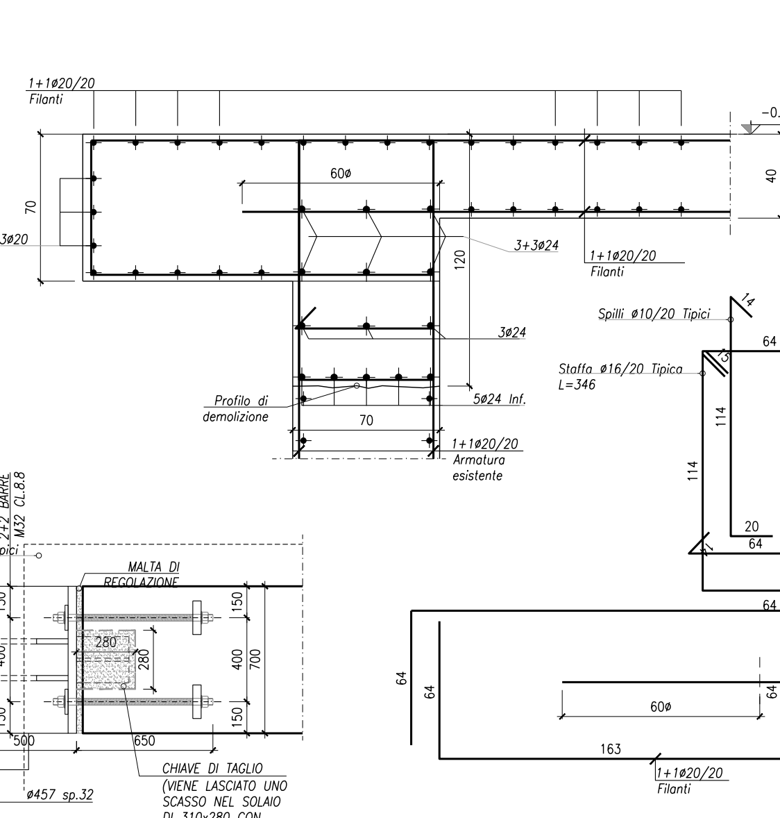
SEZIONE 3-3 SCALA 1:25
