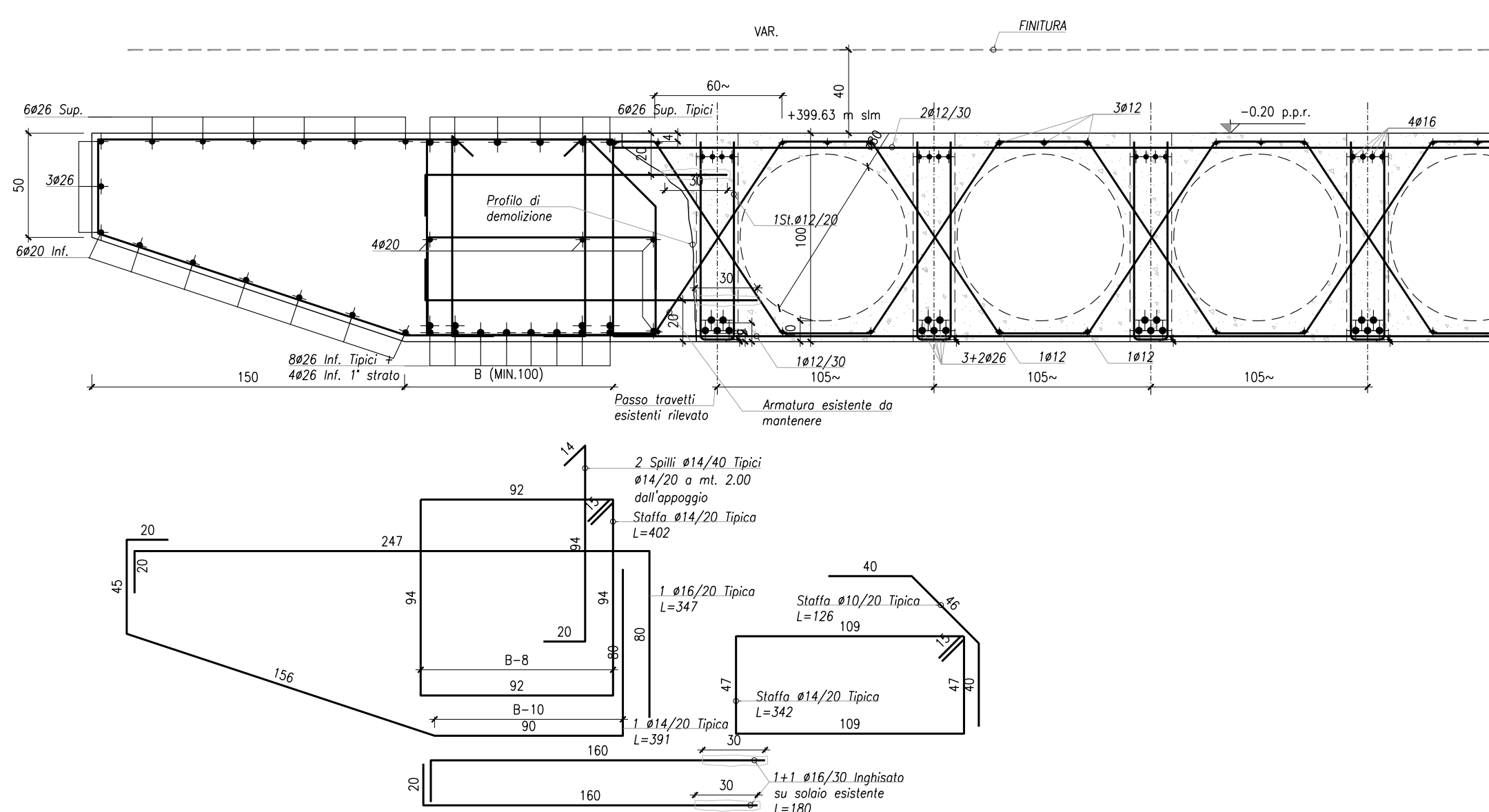
SEZIONE 1-1 SCALA 1:25
