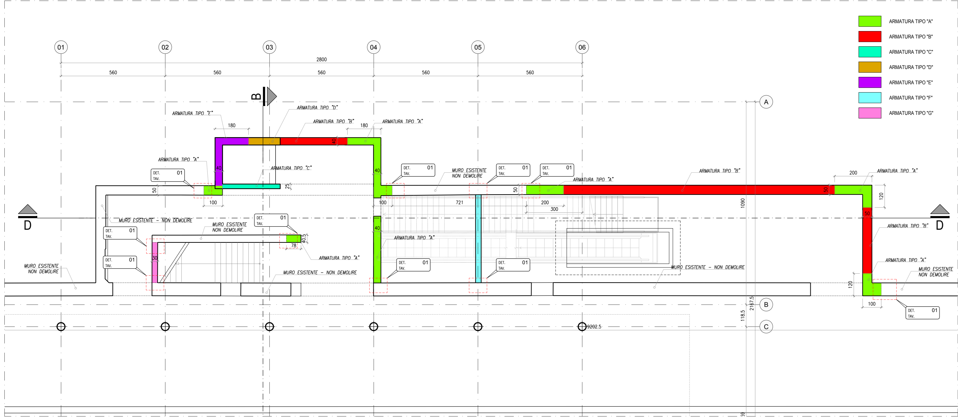
DETTAGLIO 01 SCALA 1:25 SEZIONE ORIZZONTALE
