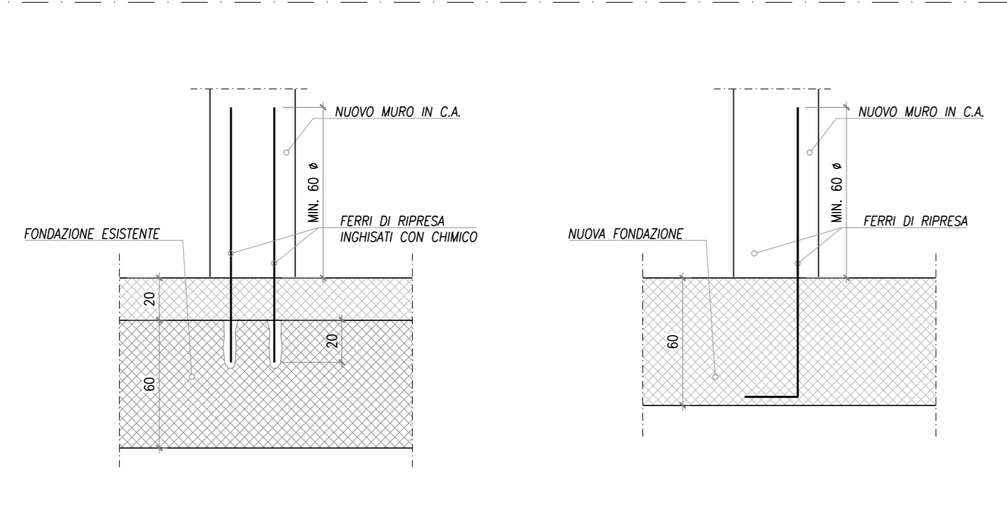
DETTAGLI RIPRESE FERRI SCALA 1:25
