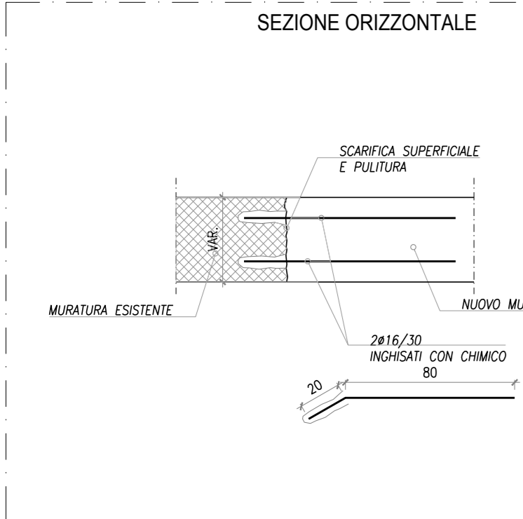
DETTAGLIO 01 SCALA 1:25 SEZIONE ORIZZONTALE
