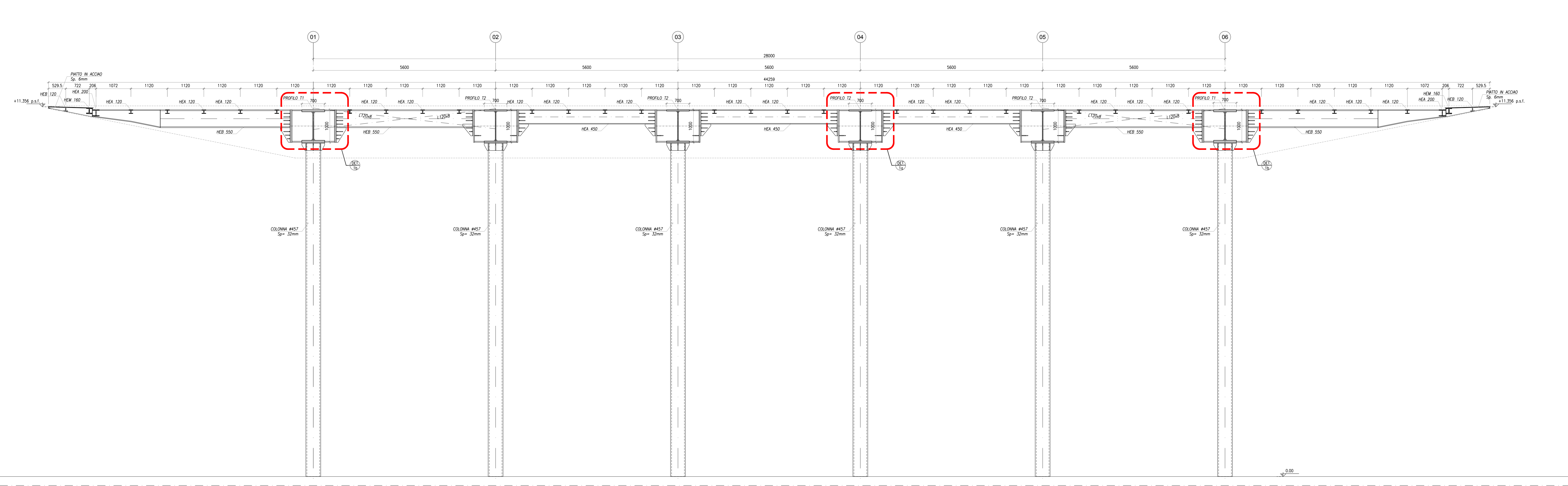
SEZIONE B-B SCALA 1:100
