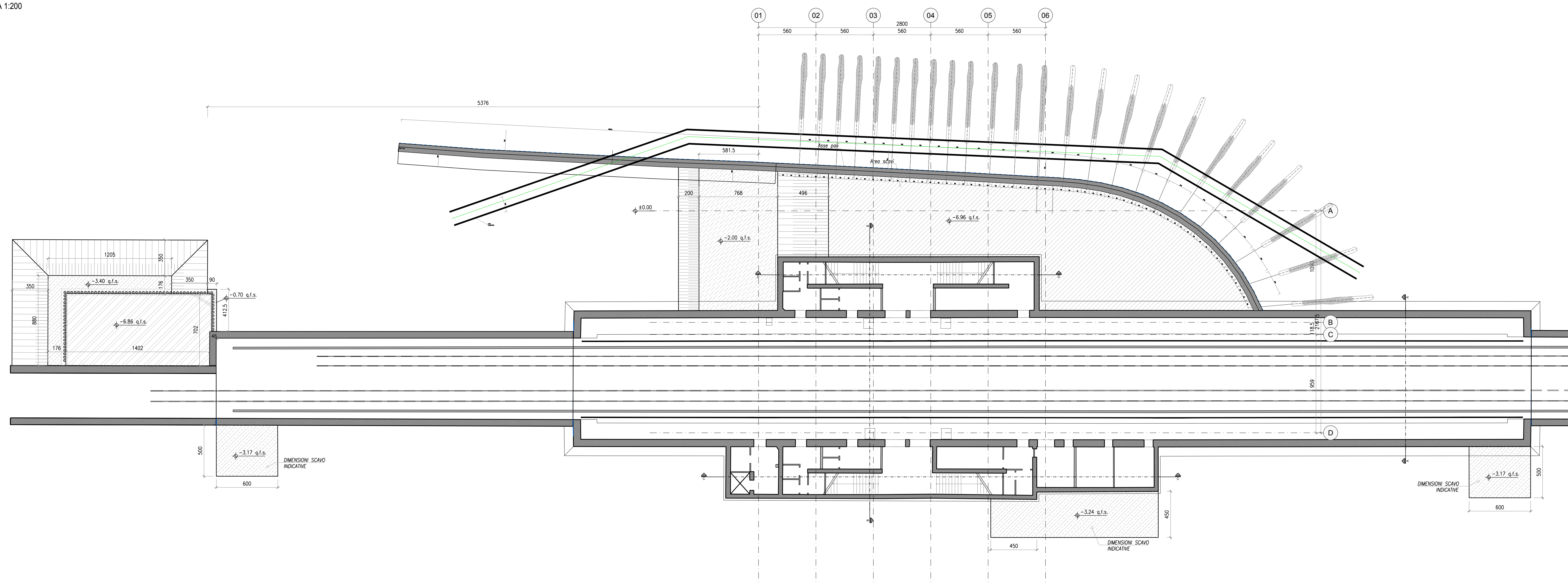
PLANIMETRIA PIANO INTERRATO - SCAVI SCALA 1:200
