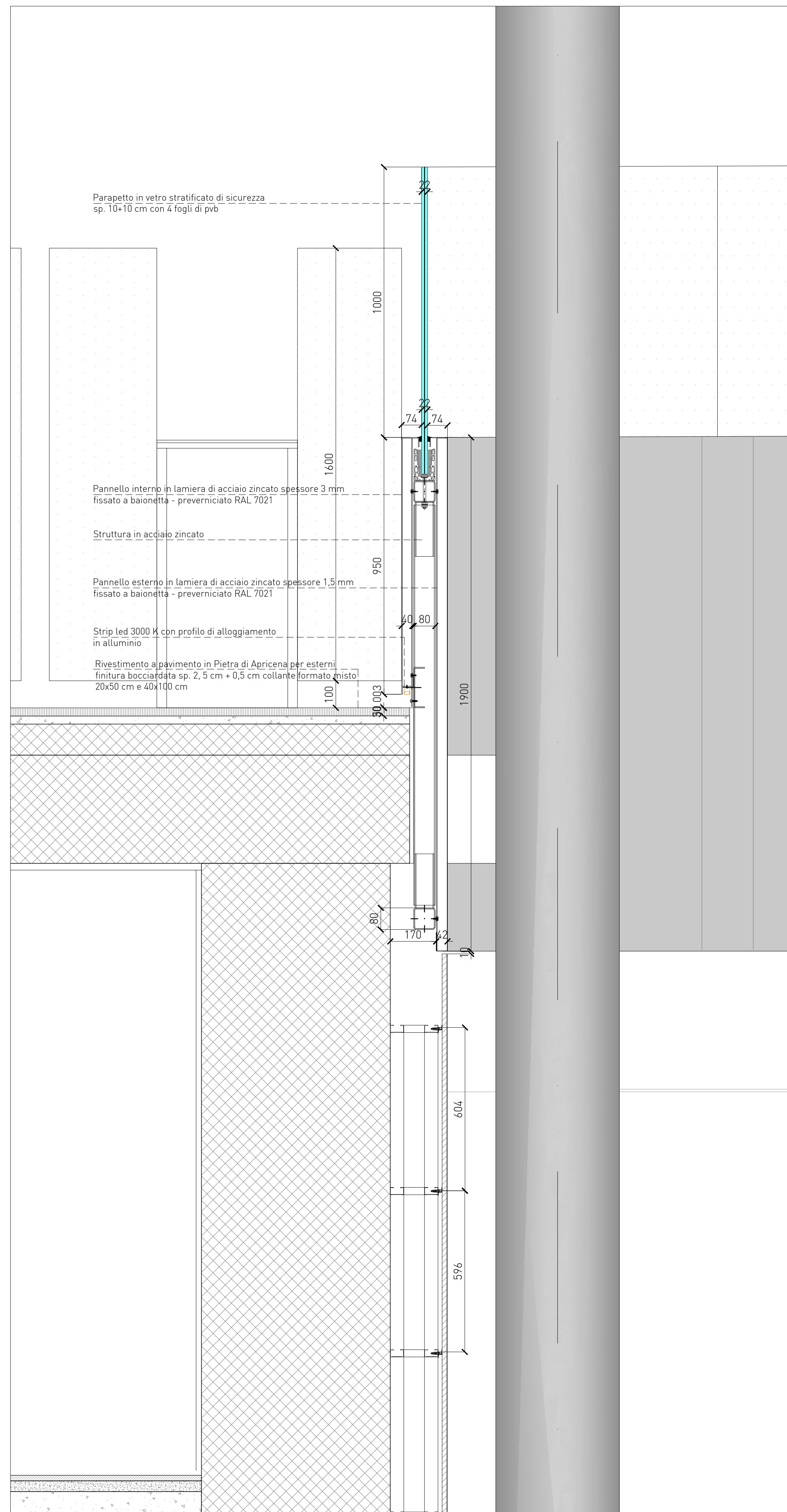
DETTAGLIO 01-PE_A.04.302_SCALA 1:10
