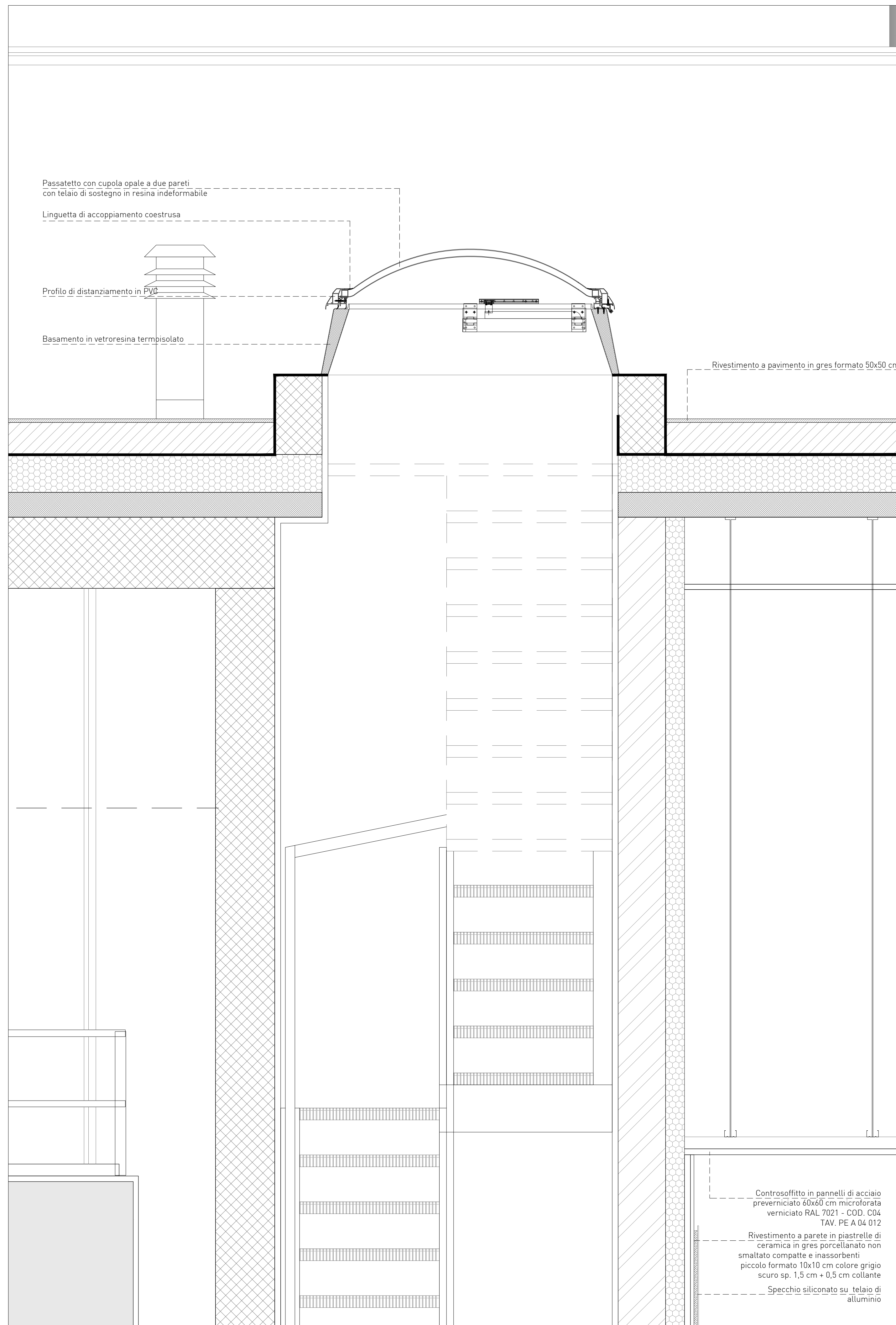
DETTAGLIO 02-PE_A.04.302_SCALA 1:10
