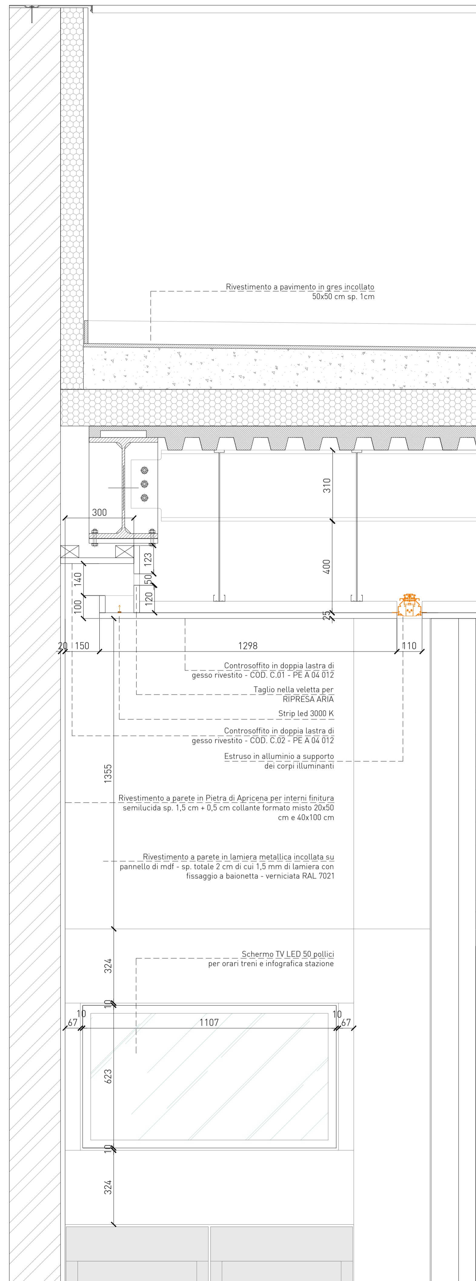
DETTAGLIO 02-PE_A.04.301_SCALA 1:10
