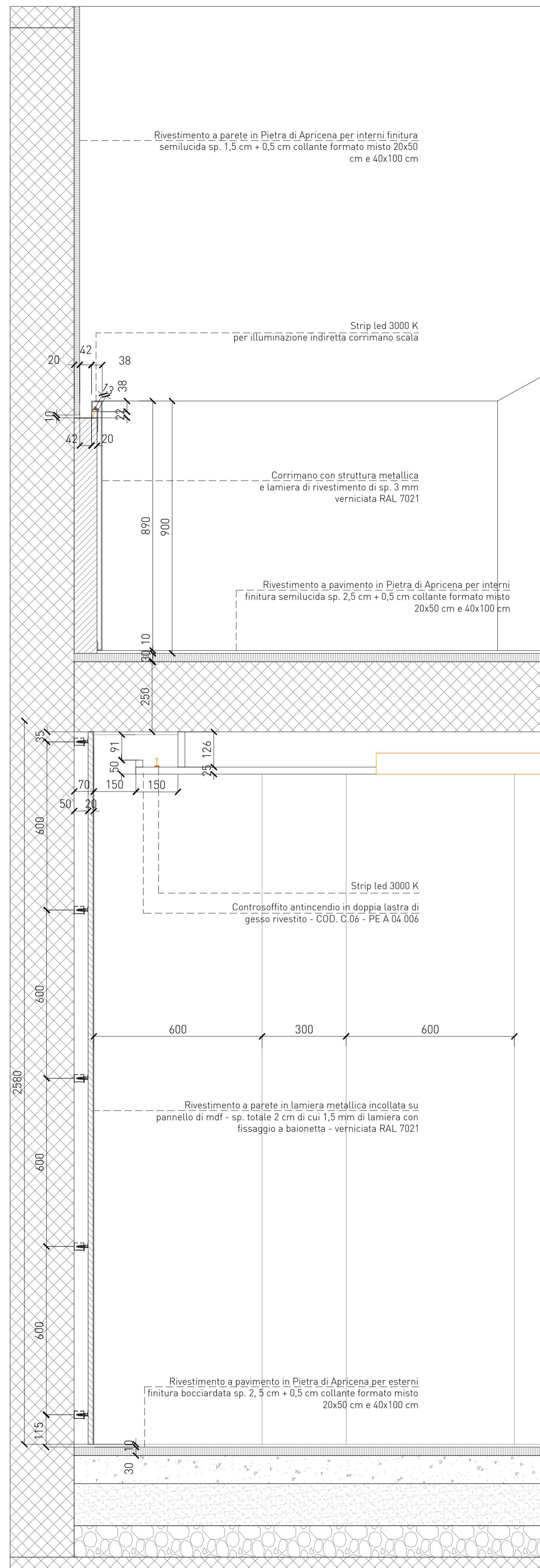
DETTAGLIO 01-PE_A.04.301_SCALA 1:10
